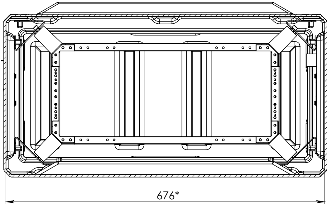
СЕЧЕНИЕ В-В МАСШТАБ 1 : 5
