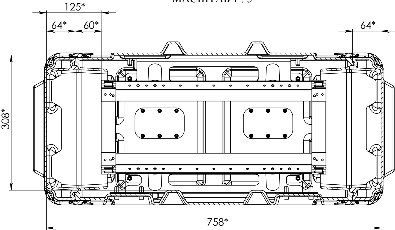
СЕЧЕНИЕ А-А МАСШТАБ 1 : 5
