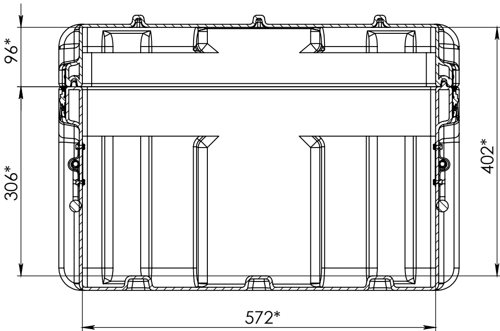
СЕЧЕНИЕ В-В МАСШТАБ 1 : 6
