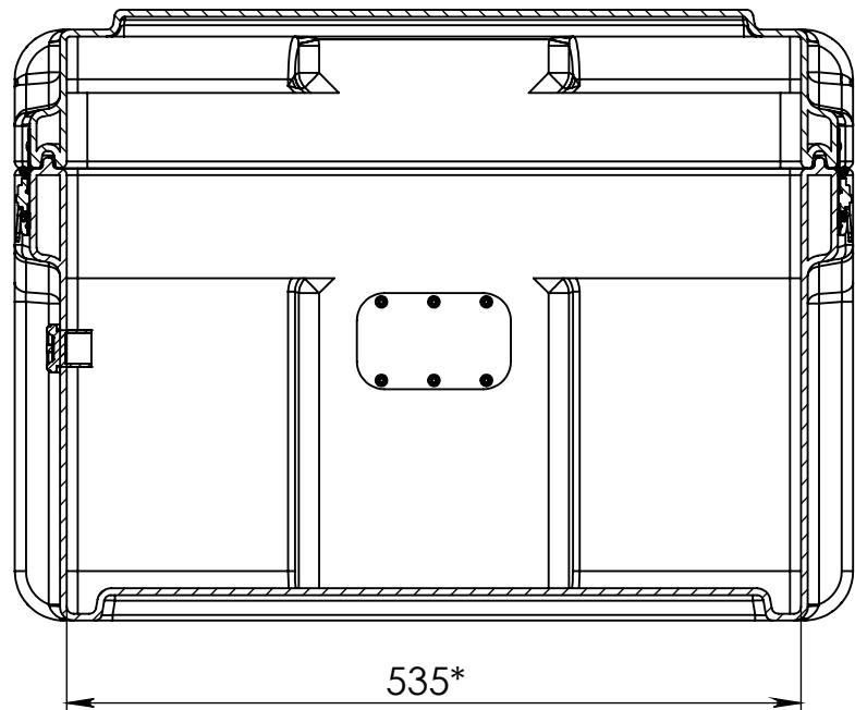
СЕЧЕНИЕ А-А МАСШТАБ 1 : 6
