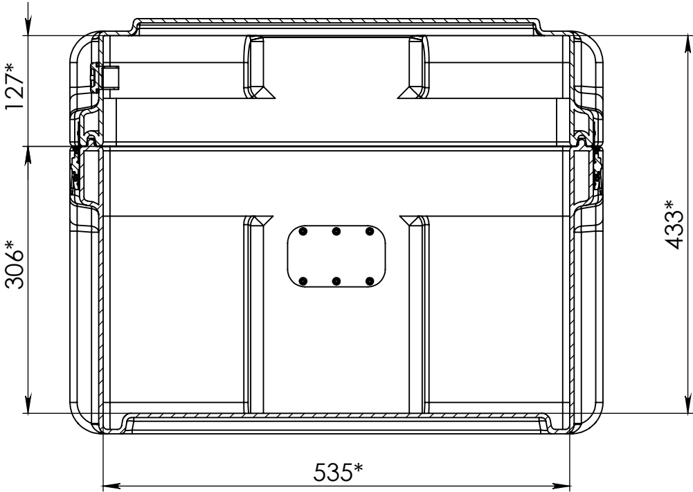
СЕЧЕНИЕ А-А МАСШТАБ 1 : 6
